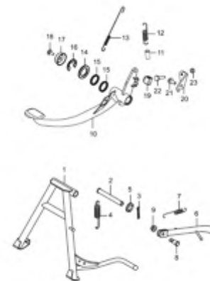
Fig. 28 STAND (P05-S270-0021)
