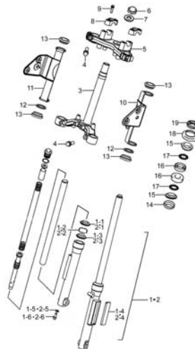
Fig. 39 STEERING STEM (X03-C400-0005)
