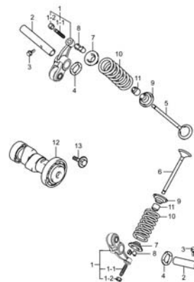
Fig. 7 CAMSHAFT-VALVE (X03-C070-0001)
