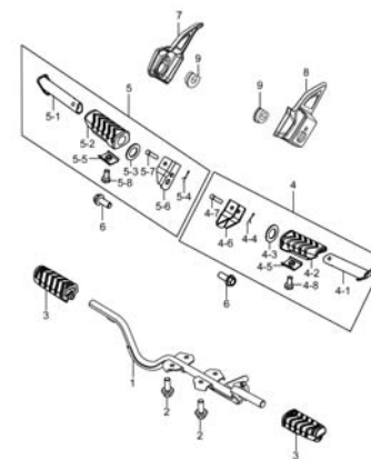
Fig. 28 FOOTREST (X03-C280-0005)
