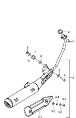
Fig. 11 MUFFLER (X03-C110-0007)
