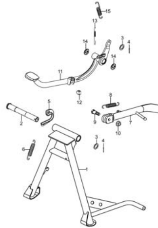
Fig. 27 STAND (P10-S270-0001)
