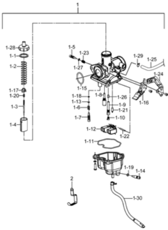
Fig. 9 CARBURETOR (P10-S090-0002)
